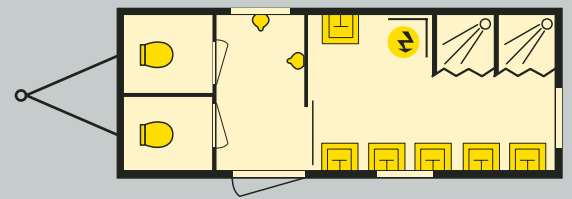
Wasch- und Toilettenwagen für 60 Mann (nach AStV)
