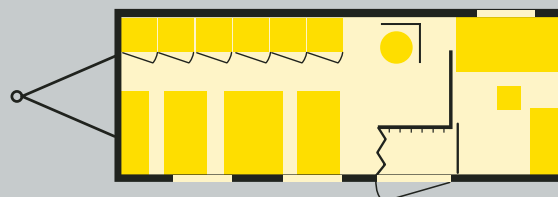
Aufenthaltswagen für 6 Mann mit Büroabteil
