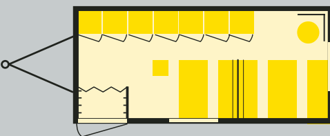
Aufenthaltswagen für 7 Mann
