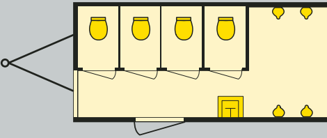
Toilettenwagen für 60 Mann (nach AStV)
