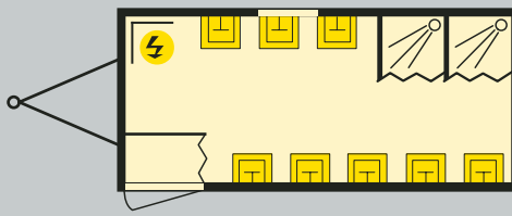
Waschwagen für 40 Mann (nach AStV)
