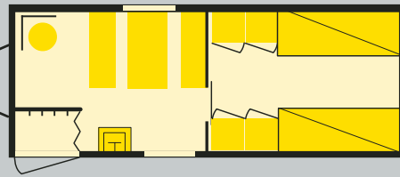
Wohn- und Schlafwagen für 4 Mann (nach AStV)
