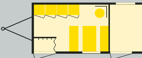
Aufenthaltswagen für 4 Mann mit Geräteabteil
