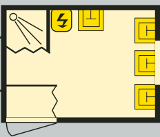
Waschwagen für 20 Mann (nach AStV)
