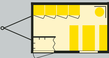
Aufenthaltswagen für 4 Mann
