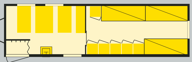
Wohn- und Schlafwagen für 6 Mann (nach AStV)
