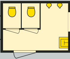
Toilettenwagen für 30 Mann (nach AStV)
