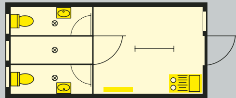
TYP C63-EURO60 Sanitär-Büro (WC's und Kleinküchenkombination)
