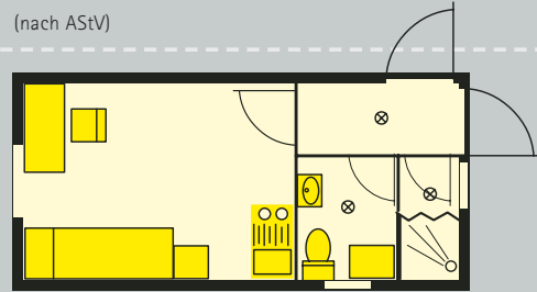
TYP C63-EURO60 Polier-/Komfortcontainer
