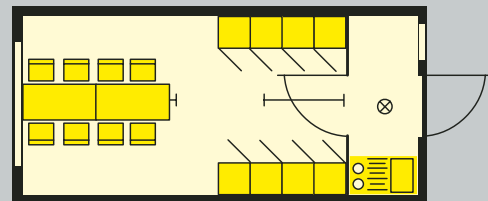
TYP C63-EURO60 Aufenthaltscontainer für 8 Mann (nach AStV)
