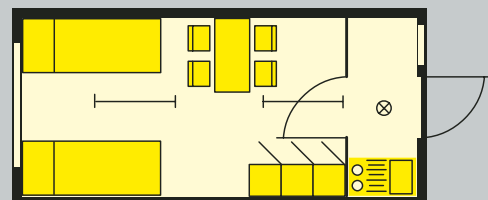
TYP C63-EURO60 Wohn- & Schlafcontainer für 3 Mann (nach AStV)
