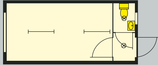
TYP C63-EURO60 mit WC-Kabine
