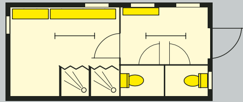
TYP C63-EURO60 Wasch- & Toilettencontainer für 25 Mann (nach AStV)
