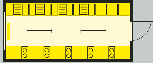
TYP C63-EURO60 Küchencontainer
