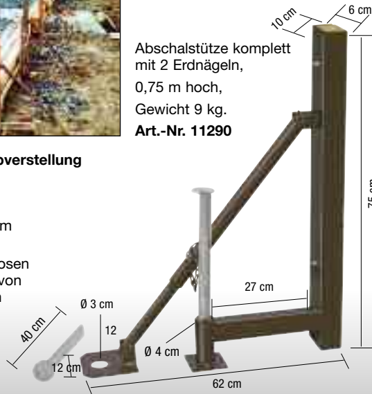
Schalhilfe zur Erstellung von Bodenplatten.
