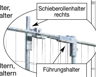
Aufbaubeispiel zweiflügelig
